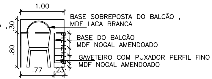
VISTA INTERNA DO BALCÃO
