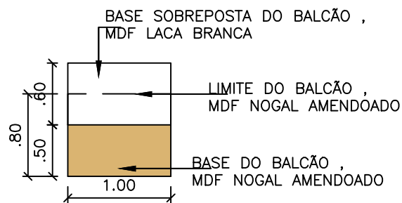
VISTA FRONTAL DO BALCÃO
