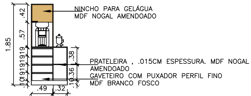
VISTA FRONTAL DO BALCÃO
