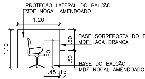
VISTA LATERAL DO BALCÃO
